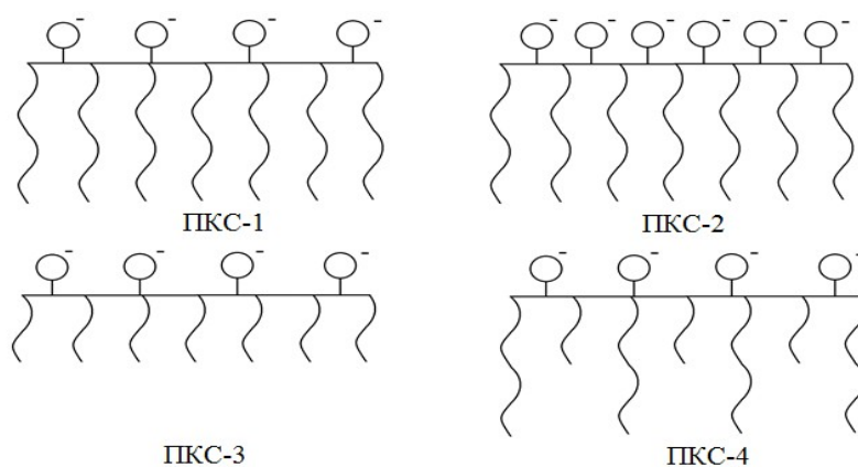
Рисунок 1 – Схема структуры поликарбоксилатных суперпластификаторов
