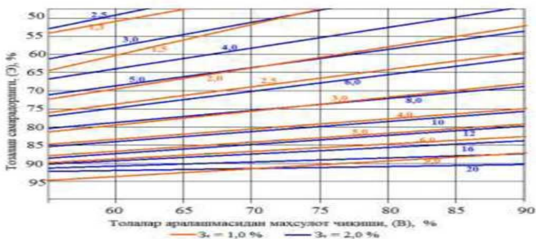
1-расм. Z_a ни B ва \mathcal{E}_k га боғлиқлигини кўрсатувчи график.
