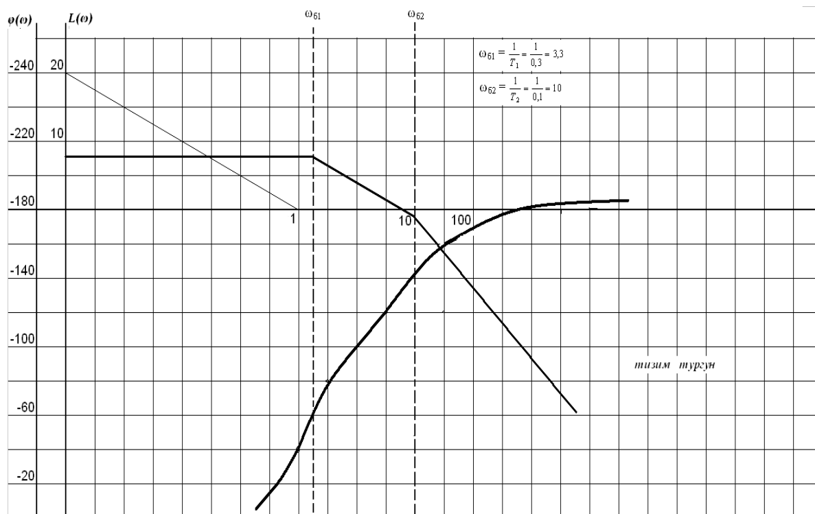
2.4-rasm. ABT ning logarifmik chastota tavsifnomalari
